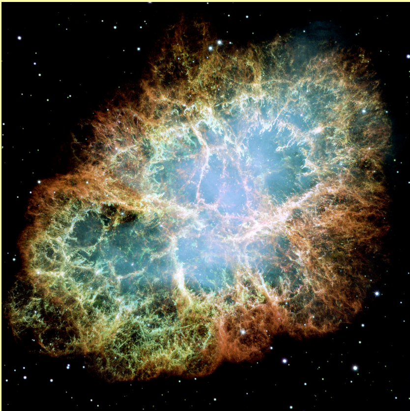
ערפילית הסרטן
